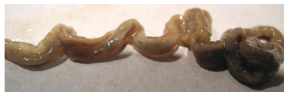
Fig 3, 4: différents stades de croissance d'un ver de corde en corps fructifère, selon l'évaluation visuelle des photographies livrées par Kerri Rivera.
